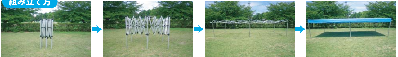
①さあ、スタート！（フレーム+天幕） ②フレームを広げます。 ③補助パイプを差し込みます。 ④天幕を被せ、支柱を伸ばせば完成。
